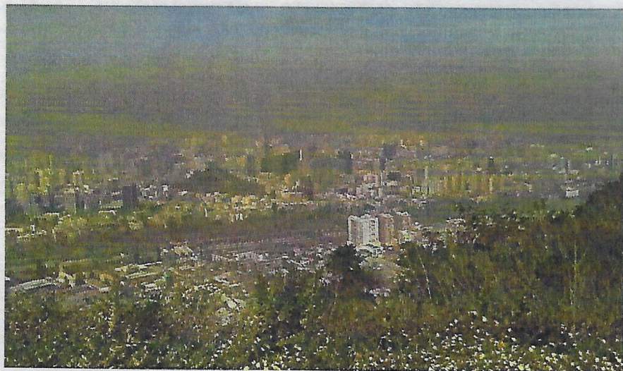
Figura 40. Con situaciones anticiclónicas, de aire encalmado, gases, humos y partículas, procedentes invariablemente de combustiones diversas y procesos industriales varios, faltos de dispersión, se acumulan y concentran a poca altura, inficionando la troposfera inferior y originando condiciones nocivas, grave peligro en ocasiones, para la salud humana. Esa fuerte presencia de sustancias contaminantes se hace patente sobre grandes urbes, intensificándose entonces en la capa geográfica su condición de manto curo ( manteau, peplos ) o boina, conocido asimismo con la expresiva denominación francesa de couchepausa (literalmente, capa sucia). En dicha circunstancia meteorológica, la peplopausa, discontinuidad que une el techo a la capa indicada, se marca con absoluta nitidez. Santiago de Chile, septiembre de 2007.
