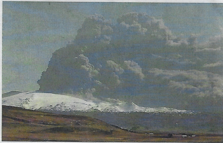
Lámina 39. Las erupciones de volcanes explosivos inyectan grandes cantidades de cenizas a la troposfera; y, con elevada concentración, originan problemas al tráfico aéreo y pueden causar, temporalmente, forzamientos radiativos negativos en el balance energético planetario. Volcán Eyjafjallajokull (Islandia) en erupción vulcaniana, abril de 2010. Fuente: exploregeography.net
